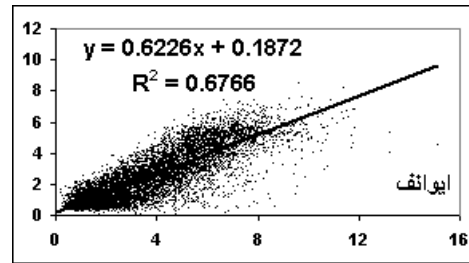
شکل 2- نمودار همبستگی بین مقادیر ET0 روزانه روش های تجربی با مقادیر ET0 روزانه روش F-P-M برای
