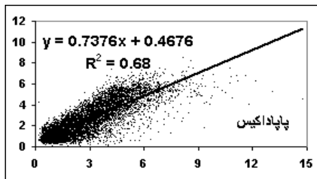
شکل 2- نمودار همبستگی بین مقادیر ET0 روزانه روش های تجربی با مقادیر ET0 روزانه روش F-P-M برای
