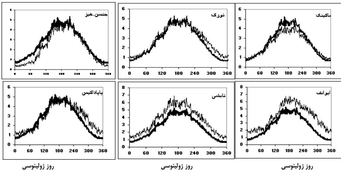
شکل 1 - نمودار بررسی نحوه تغییرات مقادیر متوسط ETo روزانه هر روز ژولینوسی معادله های تخمینی (خط باریکتر) با مقادیر متوسط ETo روزانه متناظر روش F-P-M (خط ضخیم تر) برای کل سالهای آماری (1983-2002) - ایستگاه گرگان
