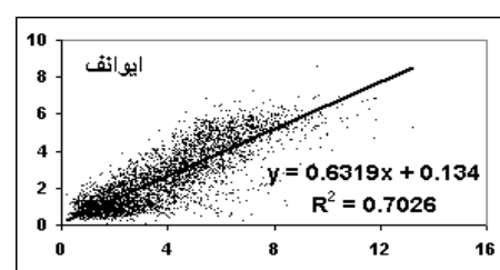
شکل 3- نمودار همبستگی بین مقادیر ET0 روزانه روش های تجربی با مقادیر ET0 روزانه روش F-P-M برای 50%
