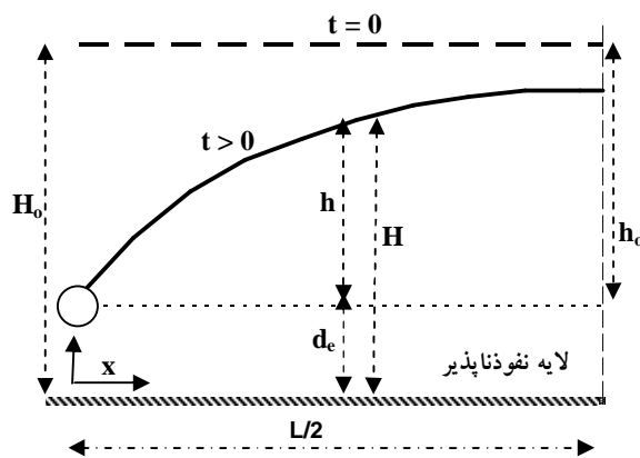
شکل 1- شماتیک و علائم توصیف کننده مسائل زهکشی زیر زمینی
