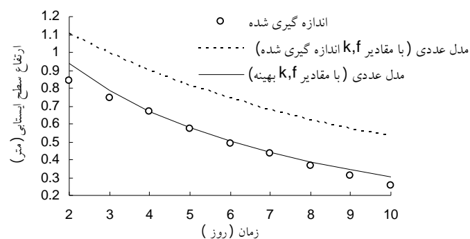
شکل 6- تغییرات زمانی مقدار ارتفاع سطح ایستابی در حد واسط دو زهکش
