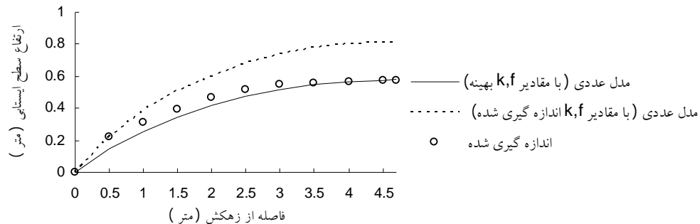
شکل 5- نیمرخ سطح ایستابی اندازه گیری شده و تخمینی از مدل عددی در زمان پنج روز از شروع زهکشی.
