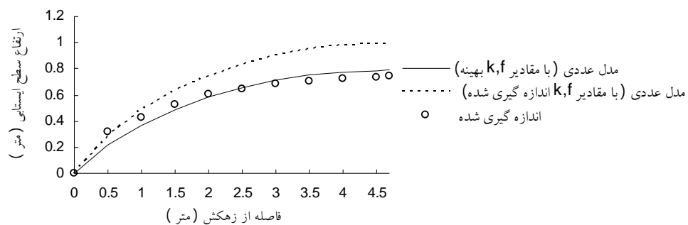
شکل 4- نیمرخ سطح ایستابی اندازه گیری شده و تخمینی از مدل عددی در زمان سه روز از شروع زهکشی.
