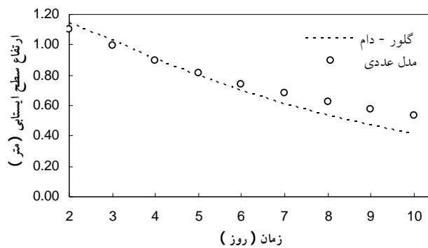
شکل 3- تغییرات زمانی ارتفاع سطح ایستابی در حد واسط دو زهکش
