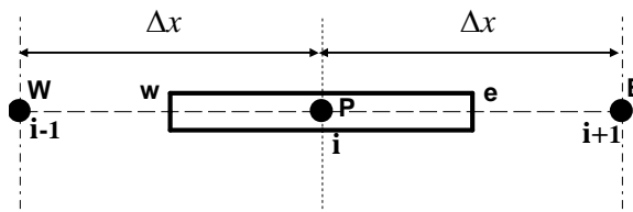
شکل 2. موقعیت حجم کنترل
