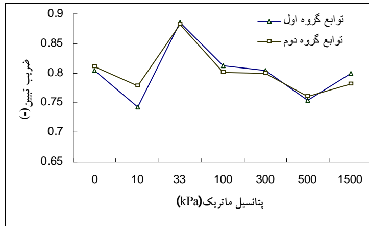
شکل 5- ضریب تبیین توابع گروه اول و دوم در پتانسیل‌های ماتریک مختلف
