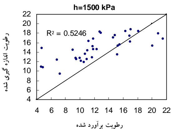
شکل 2- مقایسه همبستگی بین مقادیر رطوبتی اندازه گیری شده و برآورد شده توسط توابع پارامتریک گروه اول
