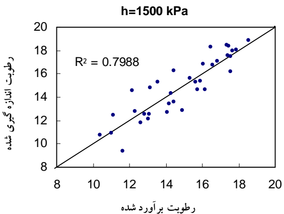
شکل 1- مقایسه همبستگی بین مقادیر رطوبتی اندازه گیری شده و برآورد شده توسط توابع نقطه‌ای گروه اول
