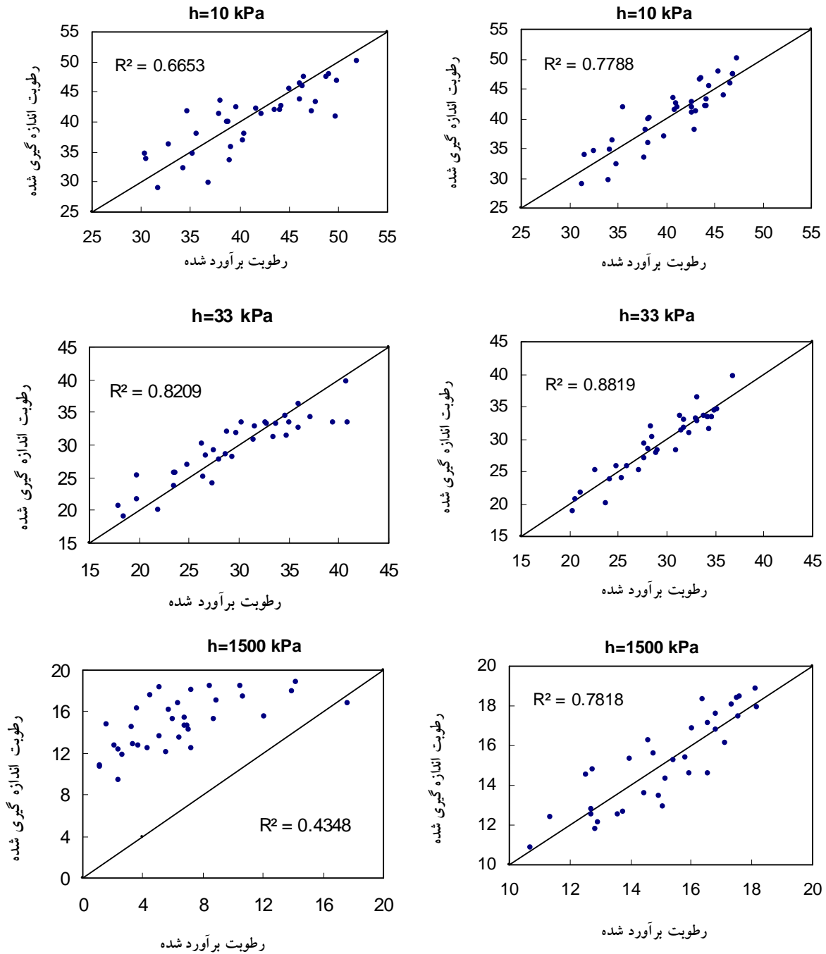
شکل 4- مقایسه همبستگی بین مقادیر رطوبتی اندازه‌گیری شده و برآورد شده توسط توابع پارامتریک گروه دوم
