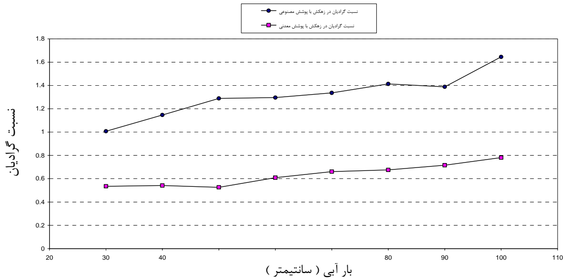
شکل ۱۰- منحنی تغییرات نسبت گرادیان با بار آبی
