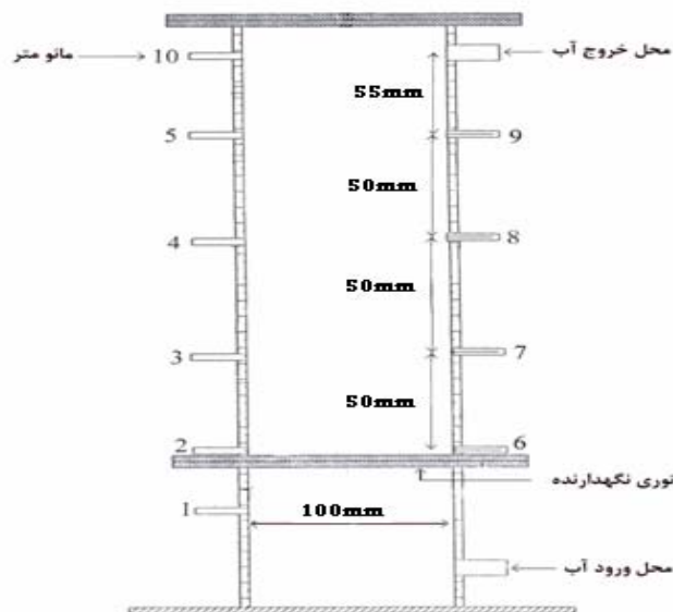
شکل ۱- دستگاه نفوذسنج شماره ۱
