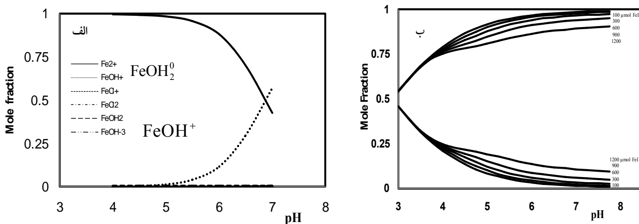
شکل ۵- (الف). توزیع گونه‌های محلول آهن (II) در غلظت ۰/۰۱ مولار NaCl مشابه با آزمایش‌های جذب سطحی و (ب). توزیع گونه‌های جذب سطحی شده آهن (II) بر اساس ضرایب ارائه شده در جدول ۲ و در غلظت ۰/۰۱ مولار NaCl
