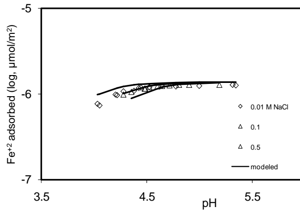
شکل ۶- هم‌دماهای جذب سطحی آهن (II) تابعی از pH تعادلی در سه سطح ۰/۱، ۰/۰۱، ۰/۱ و ۰/۵ مولار NaCl و در غلظت ۱/۹۵ گرم در لیتر گنوتایت
