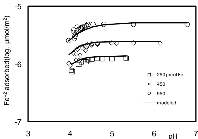
شکل ۴- هم‌دماهای جذب سطحی آهن (II) تابعی از pH تعادلی و برحسب غلظت آهن (II) جذب سطحی شده در غلظت ۰/۰۱ مولار NaCl. در این شکل نقاط داده‌های آزمایشی و خطوط پیش بینی داده‌ها بوسیله مدل CD-MUSIC بر اساس ضرایب ارائه شده در جدول ۲ را نشان می‌دهد
