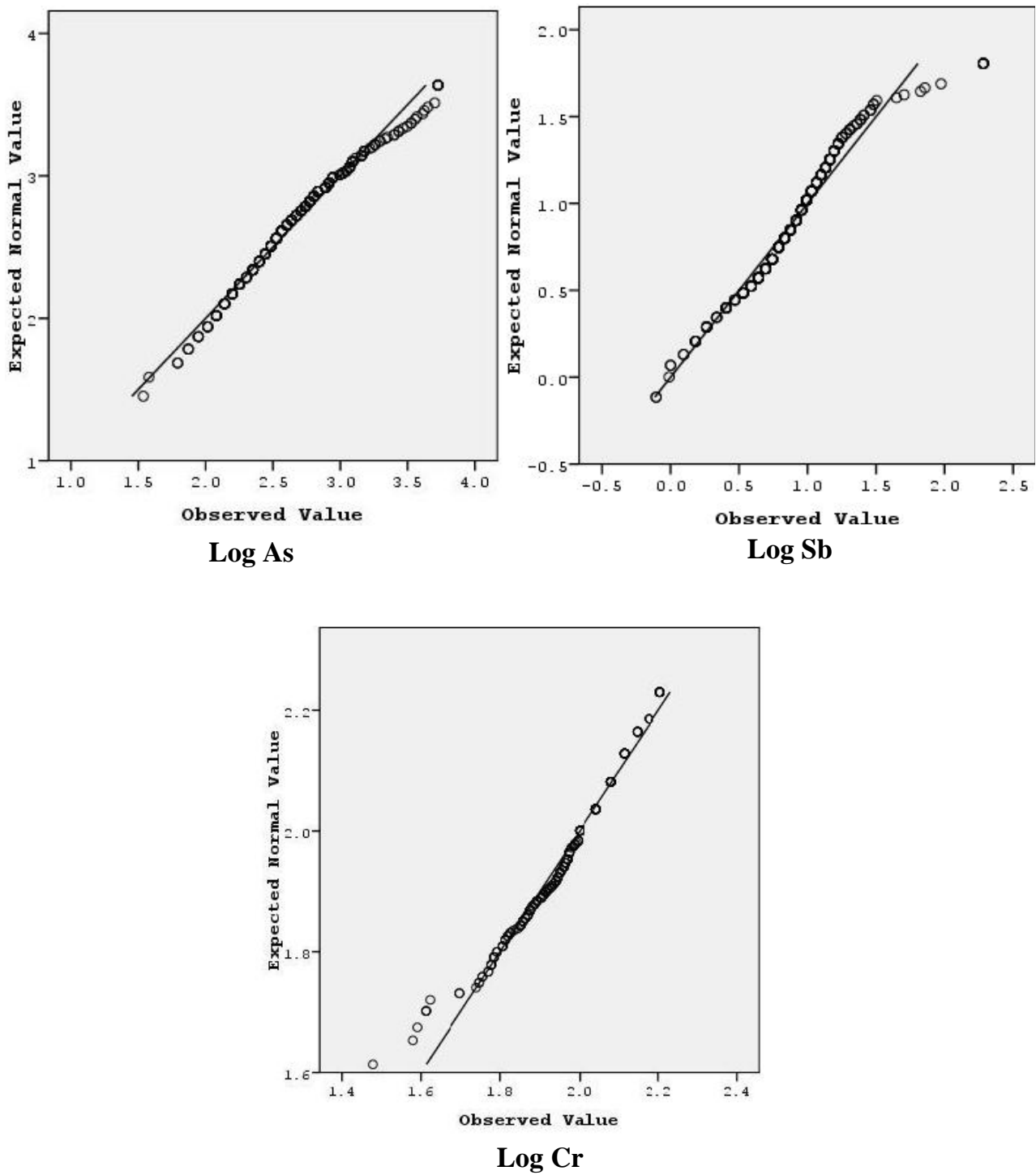
شکل ۴- نمودار Q-Q Plot لگاریتم داده های آنتیموان، آرسنیک و کروم
