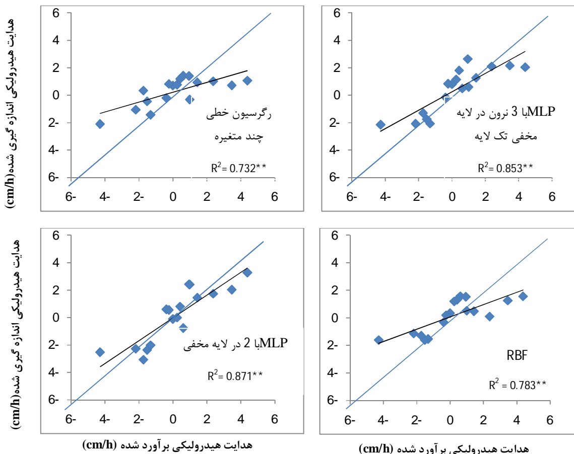
شکل 2- رابطه بین مقادیر هدایت هیدرولیکی اشباع برآورد شده با مقادیر اندازه‌گیری شده (LnKs (cm/h)) (خط آبی نشان دهنده خط 1:1 یا 45 درجه محور مختصات می‌باشد)
