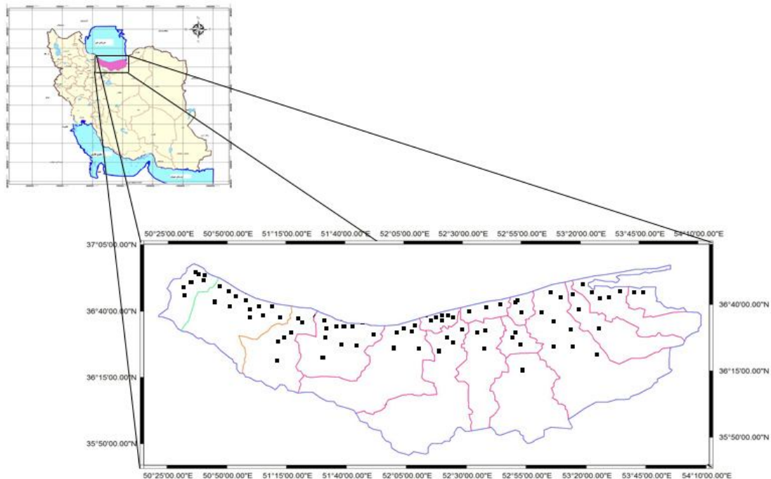
شکل 1- محل نمونه برداری داده ها در استان مازندران
