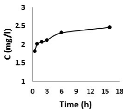
شکل 5- تغییرات غلظت پتاسیم محلول در مقابل زمان بعد از ده مرحله واجذب برای خاک‌های 2 و 9
