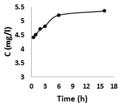
شکل 5- تغییرات غلظت پتاسیم محلول در مقابل زمان بعد از ده مرحله واجذب برای خاک‌های 2 و 9
