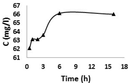
شکل 4- تغییرات غلظت پتاسیم محلول در مقابل زمان بعد از یک مرحله واجذب برای خاک‌های 2 و 9
