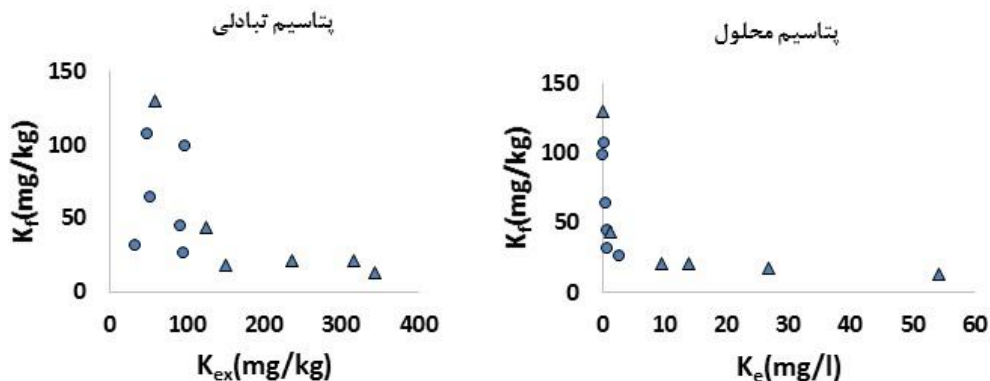
شکل 7- رابطه میزان تثبیت پتاسیم و میزان پتاسیم تبادلی (●: رس غالب اسمکتایت ▲: رس غالب ایلیت)
