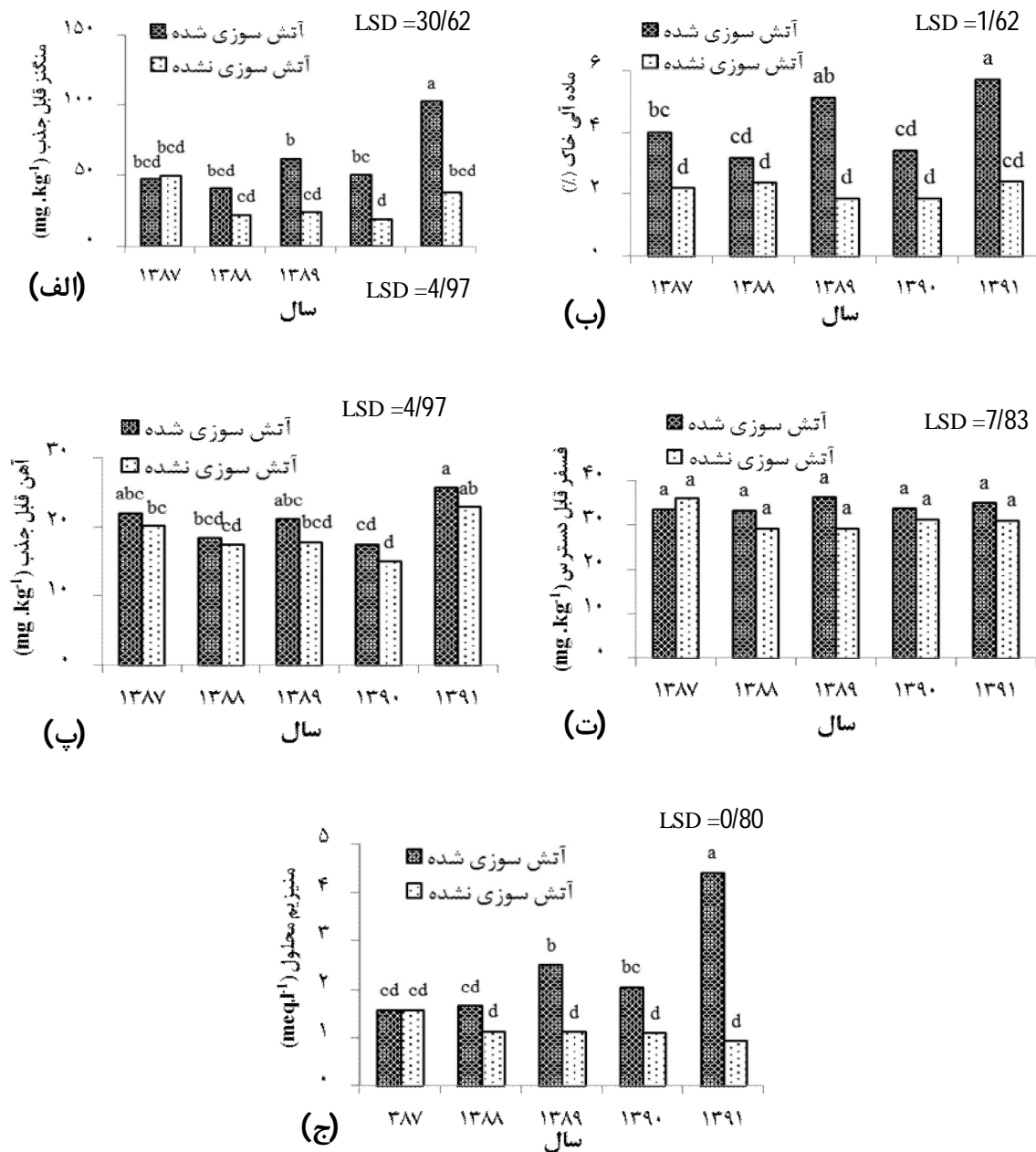
شکل 2- اثر متقابل آتش سوزی و سال بر ویژگی‌های شیمیایی خاک، (الف)-منگنز قابل استخراج با DTPA، (ب)-ماده آلی، (پ)-آهن قابل استخراج با DTPA، (ت)-فسفر قابل دسترس، (ث)- کلسیم محلول، (ج)-منیزیم محلول و (ج)-پتاسیم محلول. (میانگین‌های دارای حروف مشابه از لحاظ آماری با استفاده از آزمون LSD، در سطح احتمال 5 درصد تفاوت معنی دار ندارند).
