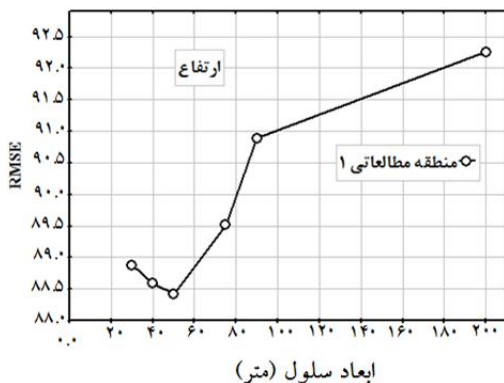
شکل 5- دقت مدل رقومی ارتفاع در ابعاد متفاوت سلول‌ها بر اساس آماره RMSE
